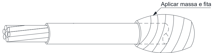
Figura 106 – Conexões e emendas – Rabicho
